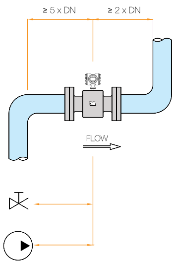
직관부 길이
