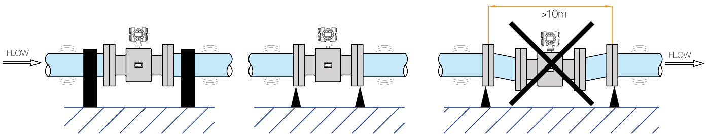
진동 방지를 위한 설치
